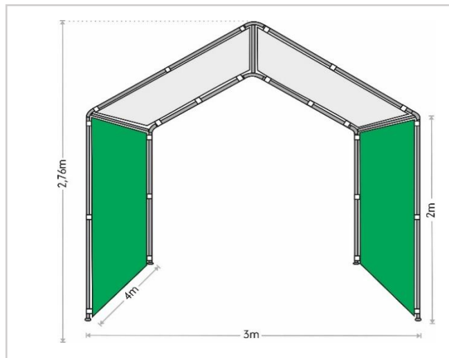
Côtes Laser 3x4m
