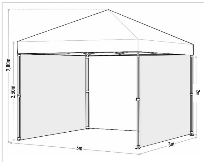
Côtes Laser 3x3m
